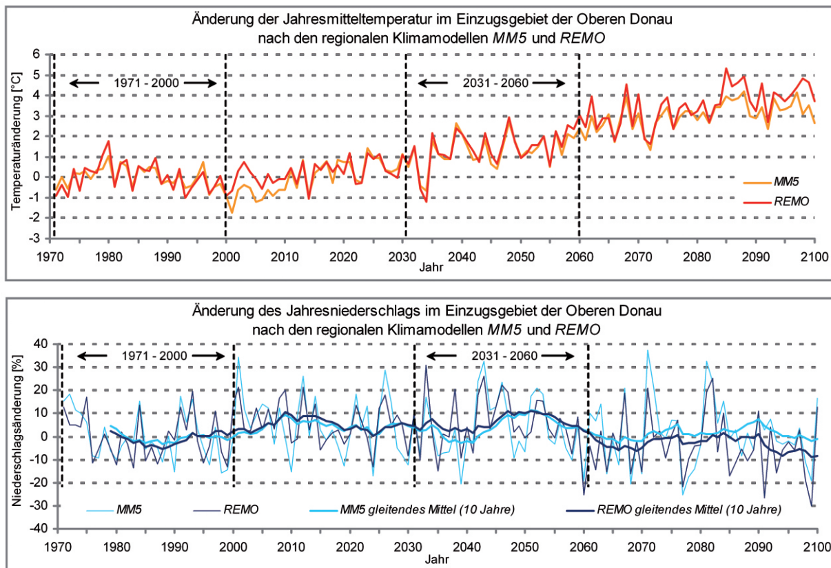
Abbildung S2.7: Abweichungen der jährlichen Mittel von Temperatur und Niederschlag zum langjährigen Mittel der Periode 1971-2000 über die Jahre 1971 bis 2100 nach Berechnungen der regionalen Klimamodelle MM5 und REMO.
