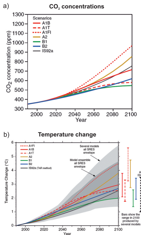
Abbildung S2.2a) Projizierter Anstieg der globalen mittleren \text{CO}_2 -Konzentration in sechs verschiedenen SRES-Szenarios; b) daraus resultierender Anstieg der globalen Mitteltemperatur (Auszug aus IPCC, 2001, Summary for Policymakers, p.14, fig.5).
