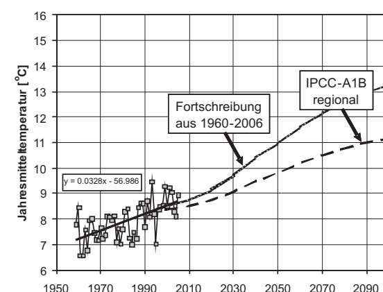
Abbildung S2.8: Verlauf des regionalen Temperaturanstiegs von 1960 bis 2100. Temperaturanstieg 1960 bis 2006 gemessen, IPCC regional für 1990 bis 2100 aus Abbildung S2.3, Fortschreibung für 1990 bis 2100 aus Kapitel 1.9.
